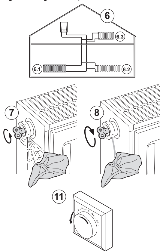
Fig.95 Degasare l'impianto
