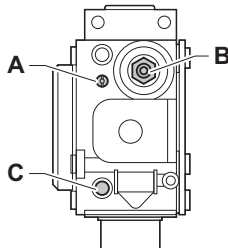
Fig.43 Punti di misurazione dell'insieme valvola gas
