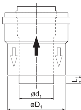
Fig.7 Dimensioni del collegamento concentrico
