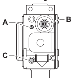
Fig.50 Assieme valvola gas
