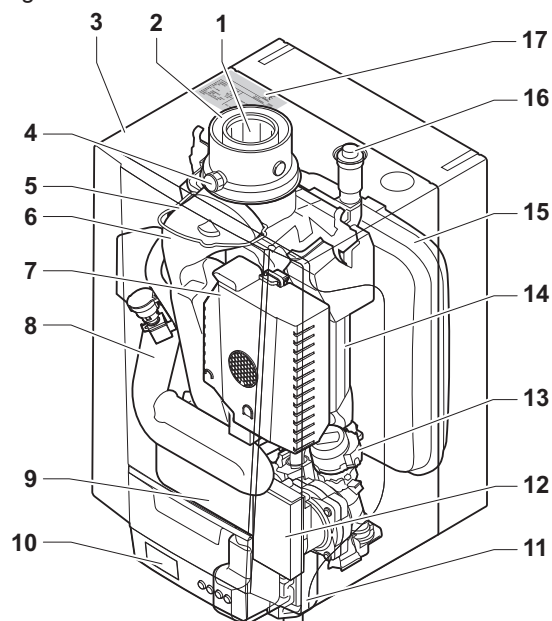
Fig.2 EMC-S 24/28 MI - 30/35 MI
