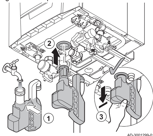
Fig.35 Riempimento del sifone
