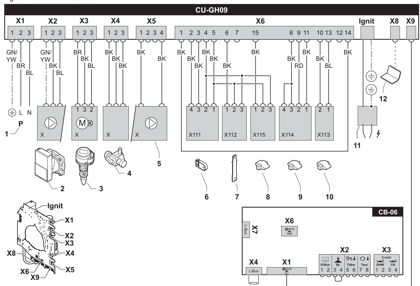
Fig.98 Schema elettrico
