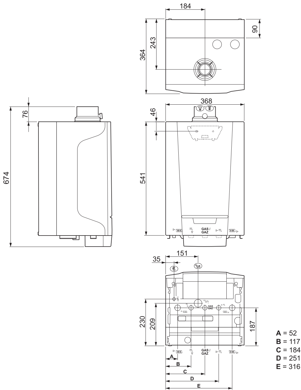
Fig.97 Dimensioni
