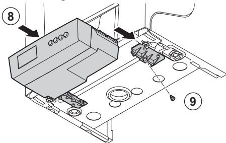
Fig.25 Montaggio della scatola dei collegamenti
