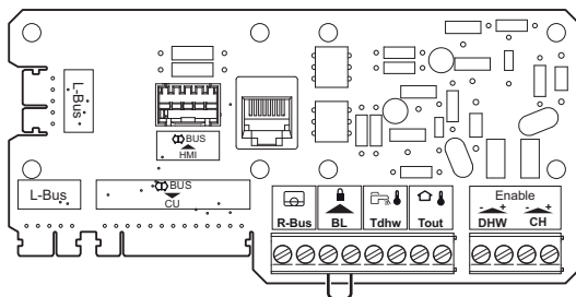
Fig.26 Scheda elettronica di controllo standard (CB-06)
