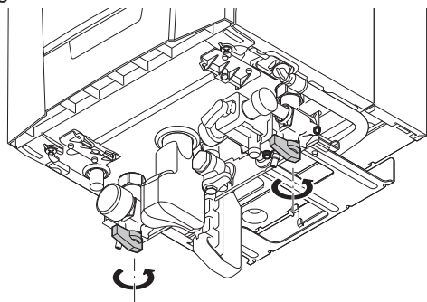
Fig.36 Valvole
