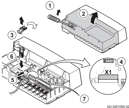
Fig.24 Accesso ai morsetti
