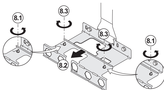
Fig.16 Estensione del telaio di montaggio
