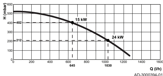
Fig.99 EMC-S 24
