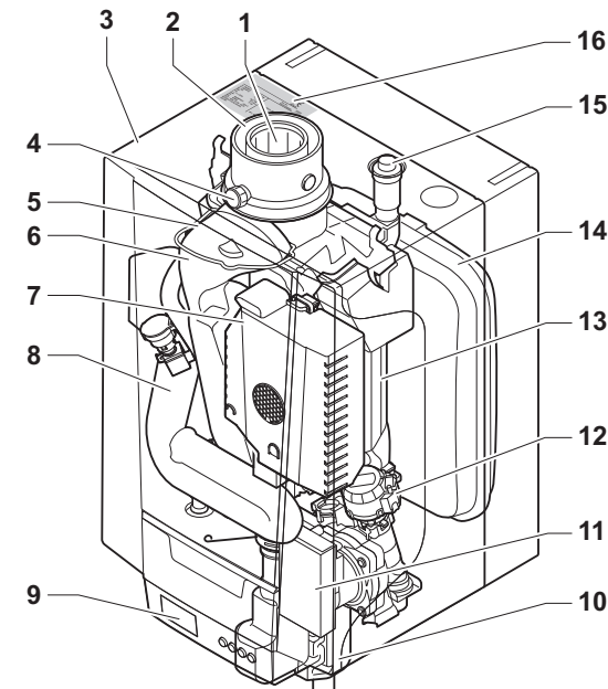
Fig.1 EMC-S 24 - 34
