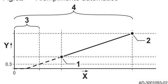
Fig.62 Riempimento automatico
