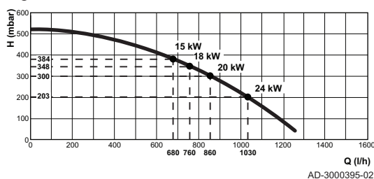
Fig.100 EMC-S 24/28 MI
