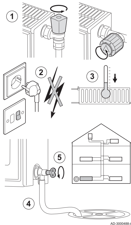
Fig.96 Svuotamento dell'impianto
