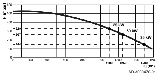
Fig.101 EMC-S 34 - 30/35 MI
