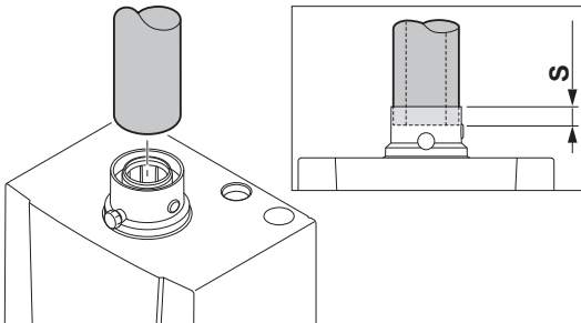
Fig.21 Collegamento dell'ingresso aria e dell'uscita fumi
