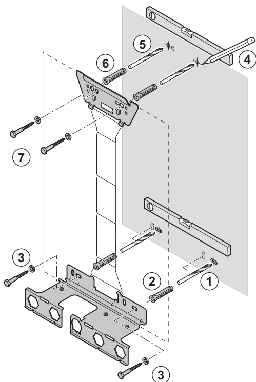
Fig.16 Estensione del telaio di montaggio
