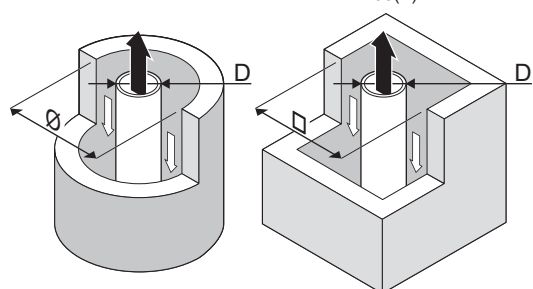
Fig.4 Dimensioni minime della canna fumaria o del condotto C 93(X)
