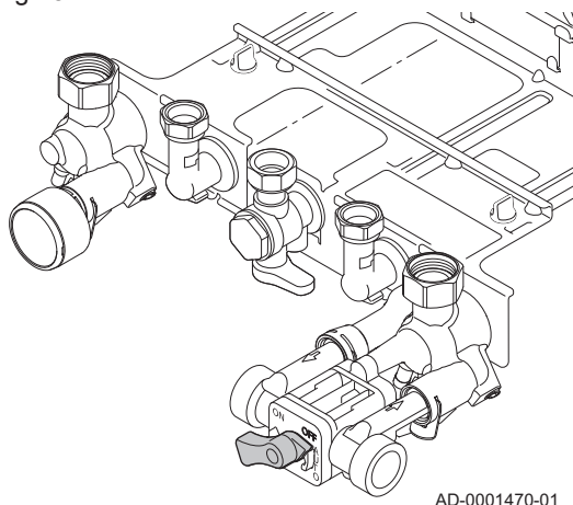
Fig.19 Montaggio della caldaia
