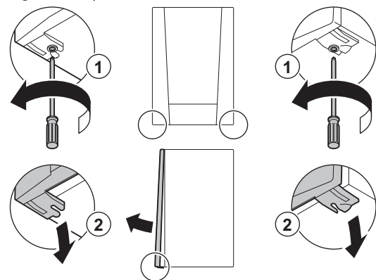
Fig.67 Apertura della caldaia
