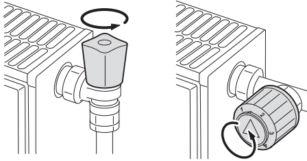
Fig.56 Aprire le valvole del radiatore
