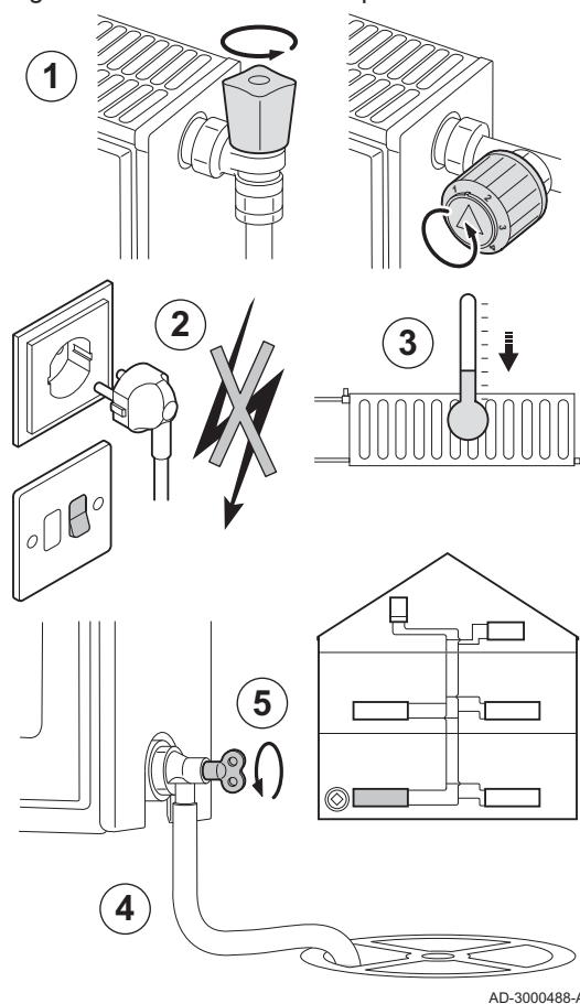
Fig.63 Svuotamento dell'impianto
