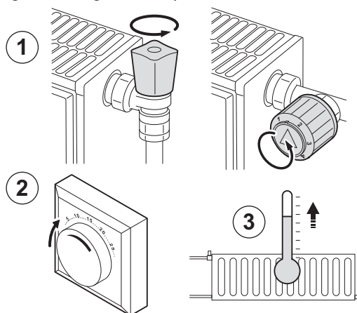
Fig.60 Degasare l'impianto
